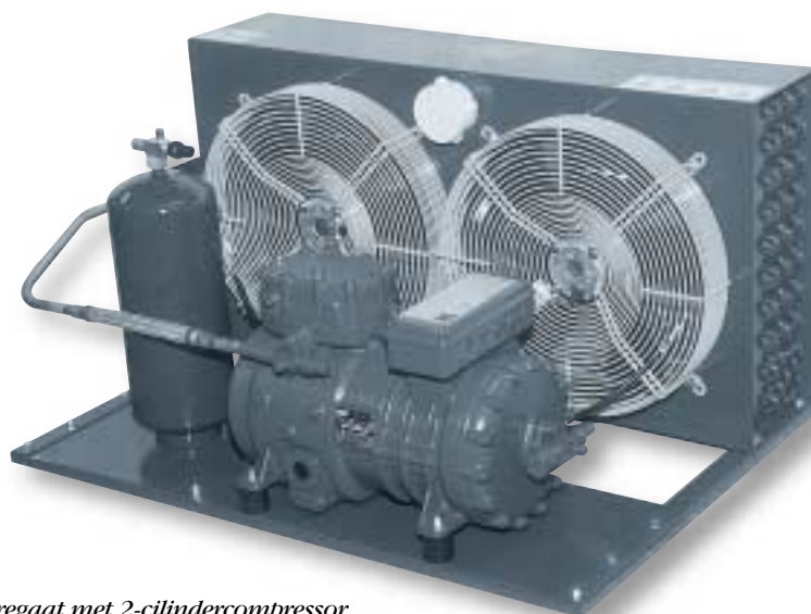
Frascold aggregaat met 2-cilindercompressor en een condensor met 2 ventilatoren.
